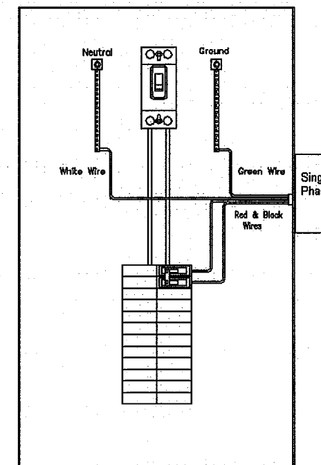
Localización del supresor Con Interruptor de SPD
